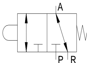
Figure 5: détail vanne 3/2.
