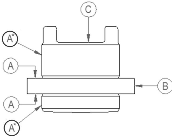
Abbildung 9 – HOB3 Nockenabtriebsbuchse, wichtige Flächen
