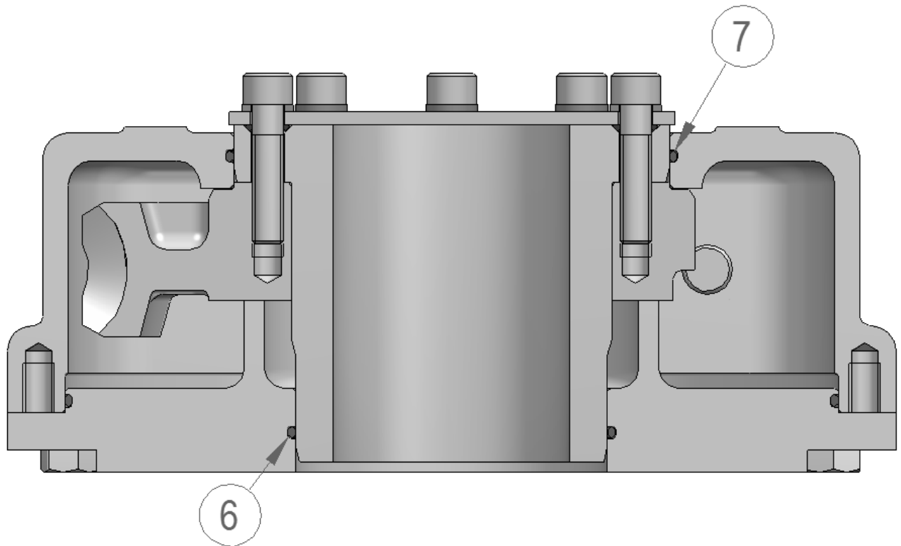
Abbildung 3 - O-Ring Überprüfung
