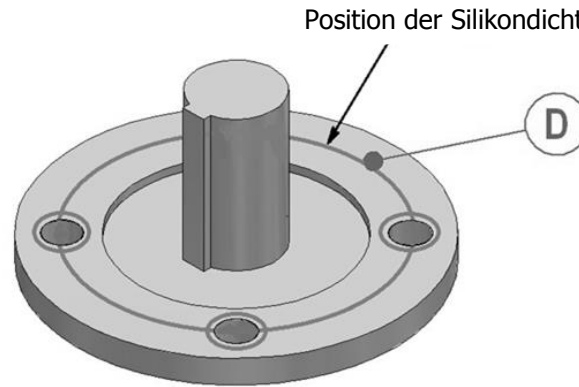
Abbildung 11 - Abdichtung des Armaturenflansches
