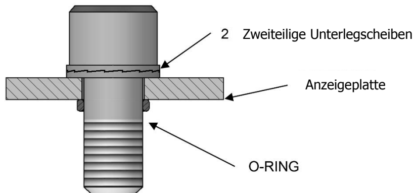
Abbildung 4 – Zweiteilige Unterlegscheiben und O-Ring Gestaltung
