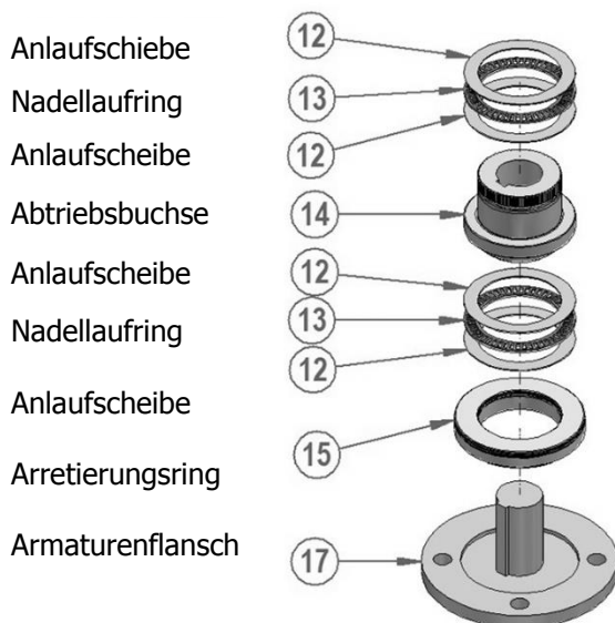
Abbildung 12 – Aufbau auf die Armaturenwelle
