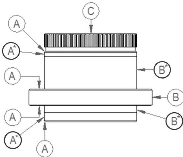
Abbildung 8 – Kerbverzahnte Ausgangsbuchse, wichtige Flächen
