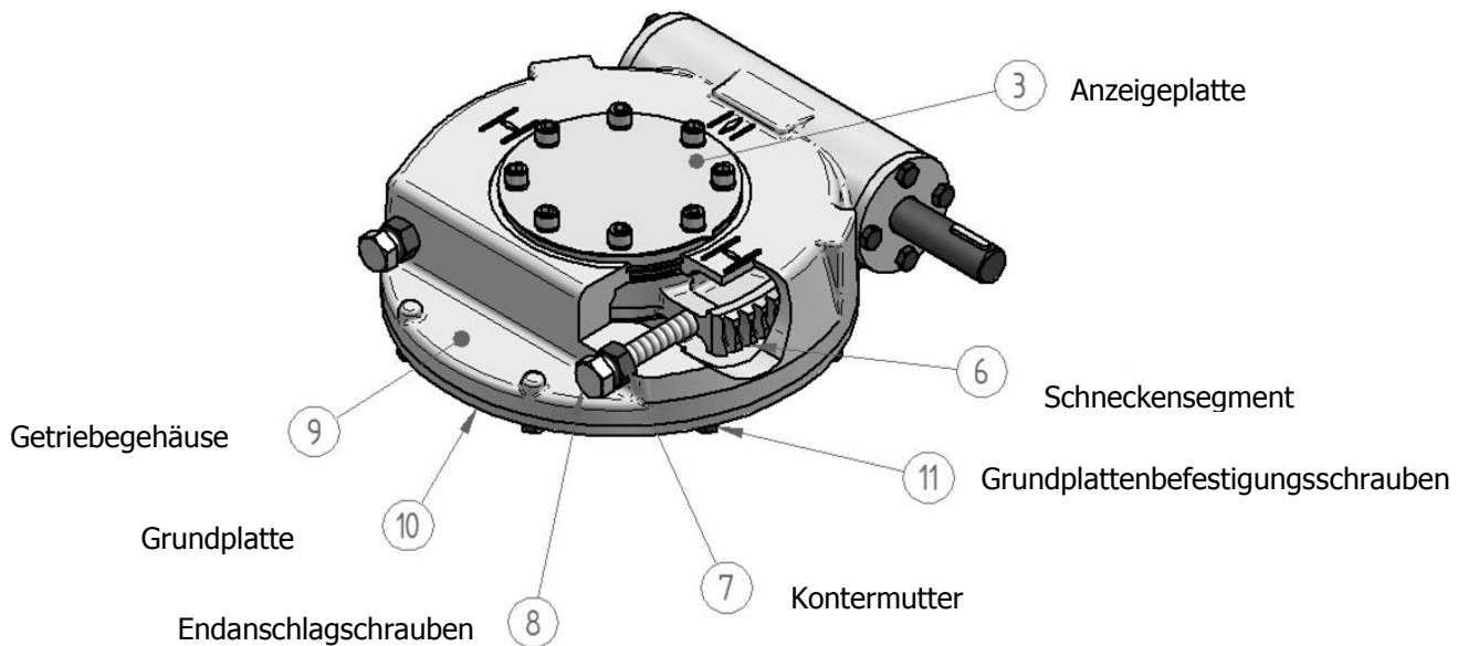
Abbildung 6 – Einstellung der Getriebeendanschläge
