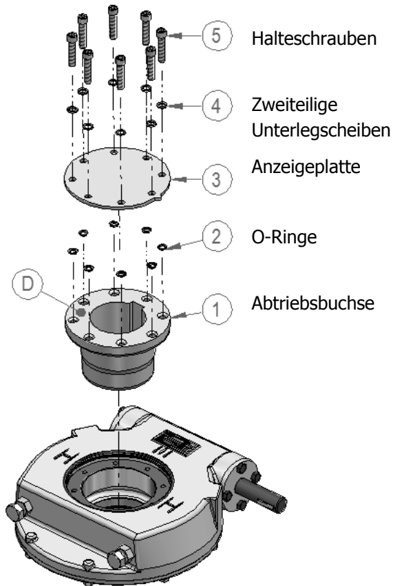
Abbildung 1 - Montage der Abtriebsbuchse
