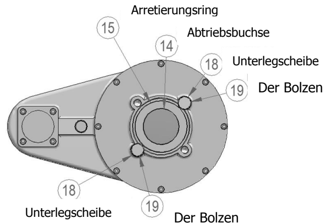
Abbildung 10 - Befestigen der Arretierungsring
