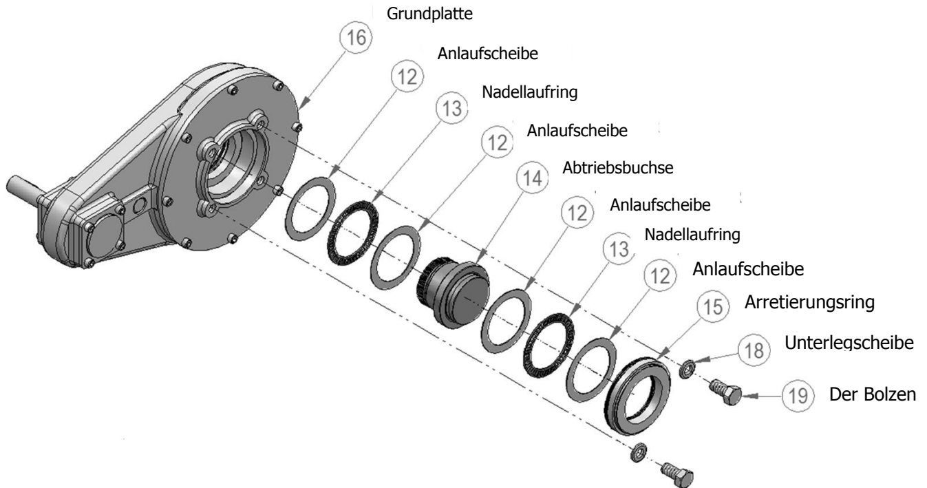
Abbildung 7 – IB / IS Zusammenbau die Abtriebsbuchse
