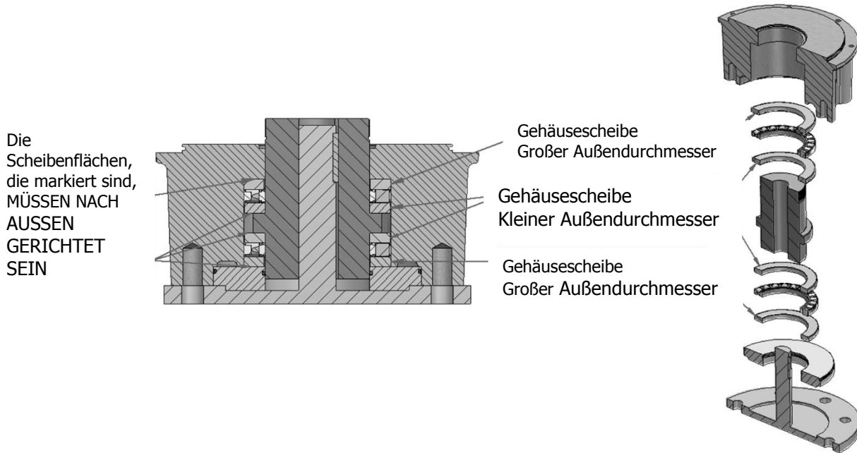
Abbildung 14 – Montage mit Zylinderrollenlager
