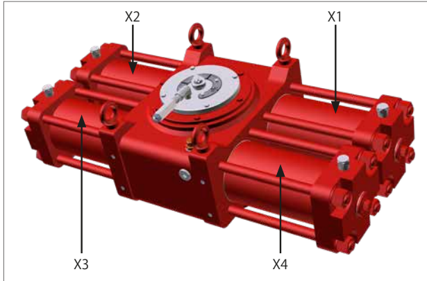
図 12.5 RH/D4 (本体サイズ090、105、125、145、155、185、225、250、280)のシリンダーの識別図
