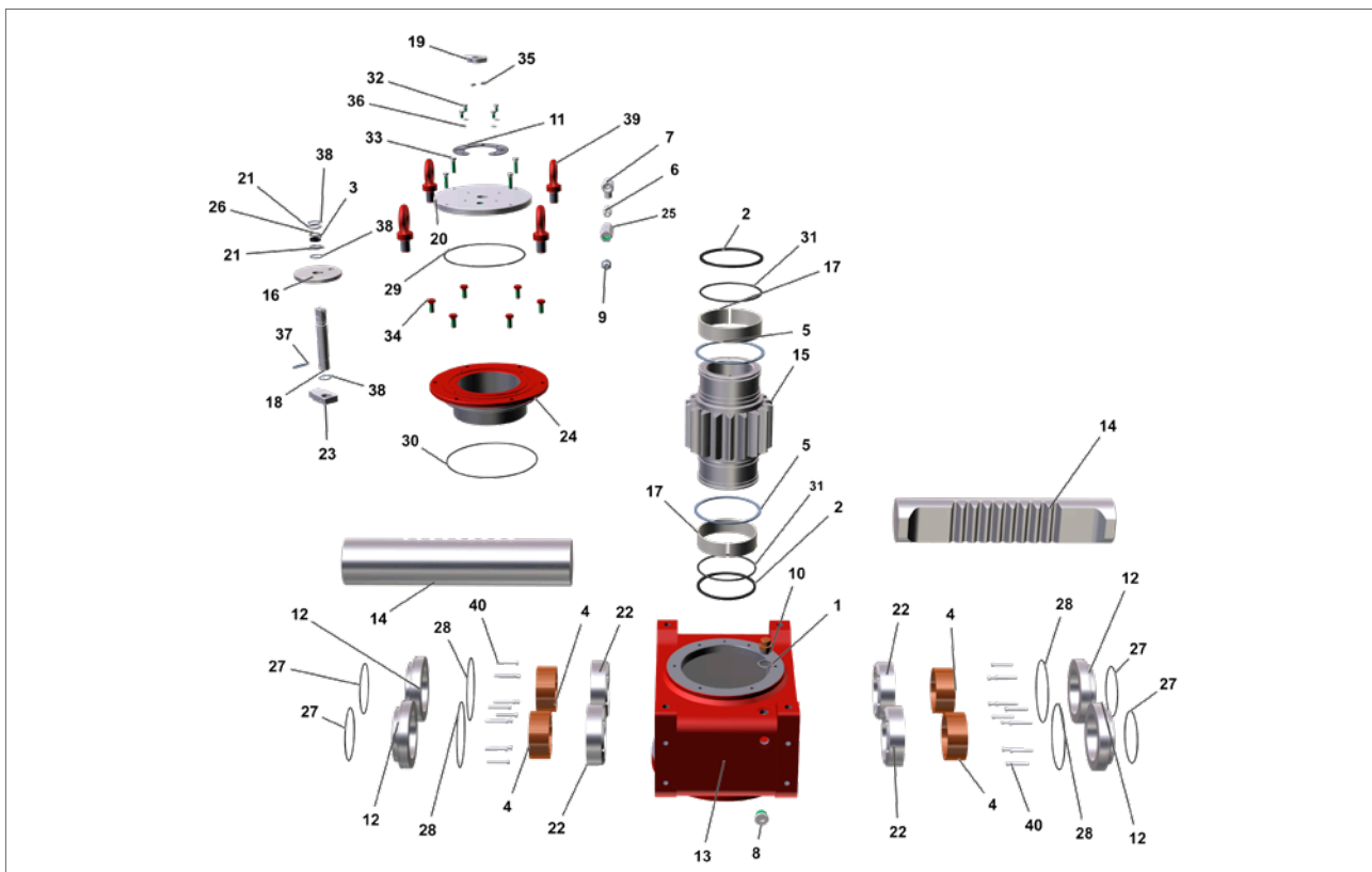
図 17.3 RH/D4複動アクチュエータ (シリンダー4個タイプ) の中央ボディ
